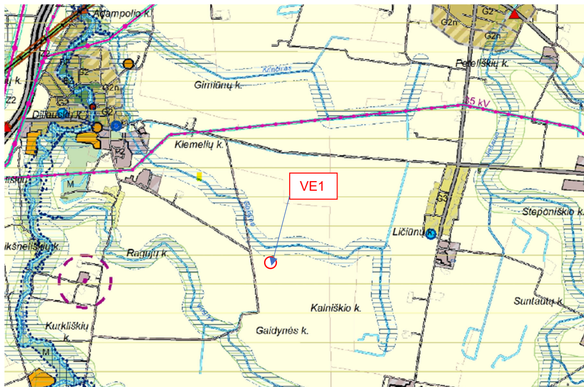
2 pav. Planuojamo projektuoti statinio vieta bendrojo plano pagrindinio brėžinio kontekste.
