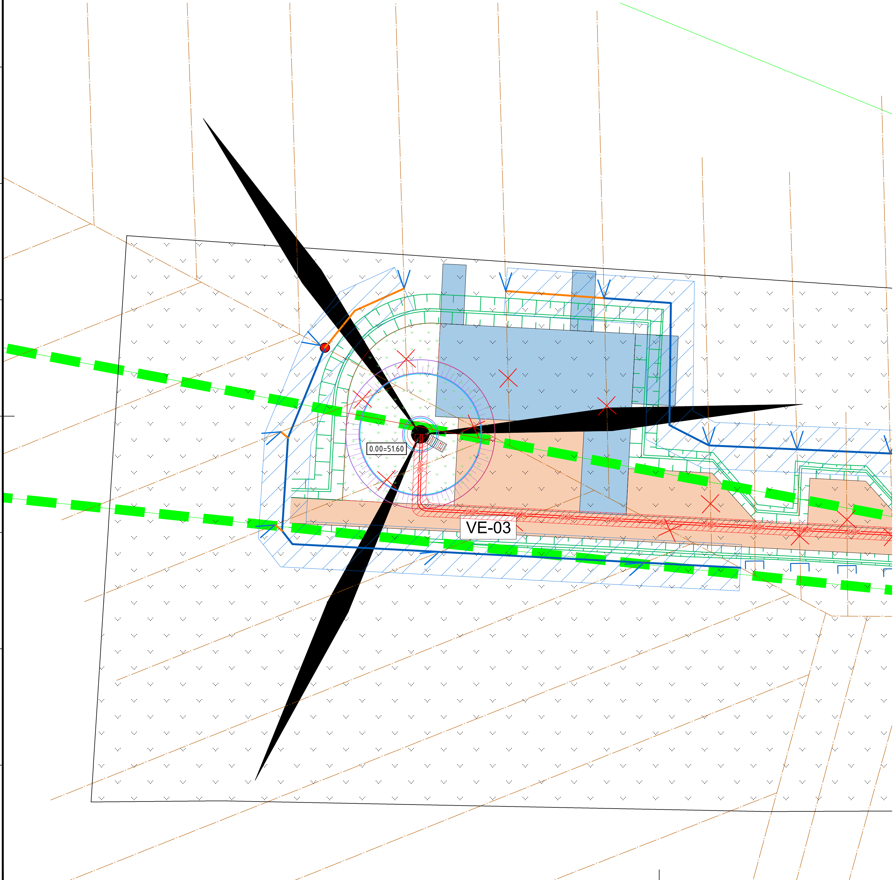
Sklypo inžinerinių tinklų planas M1:500
