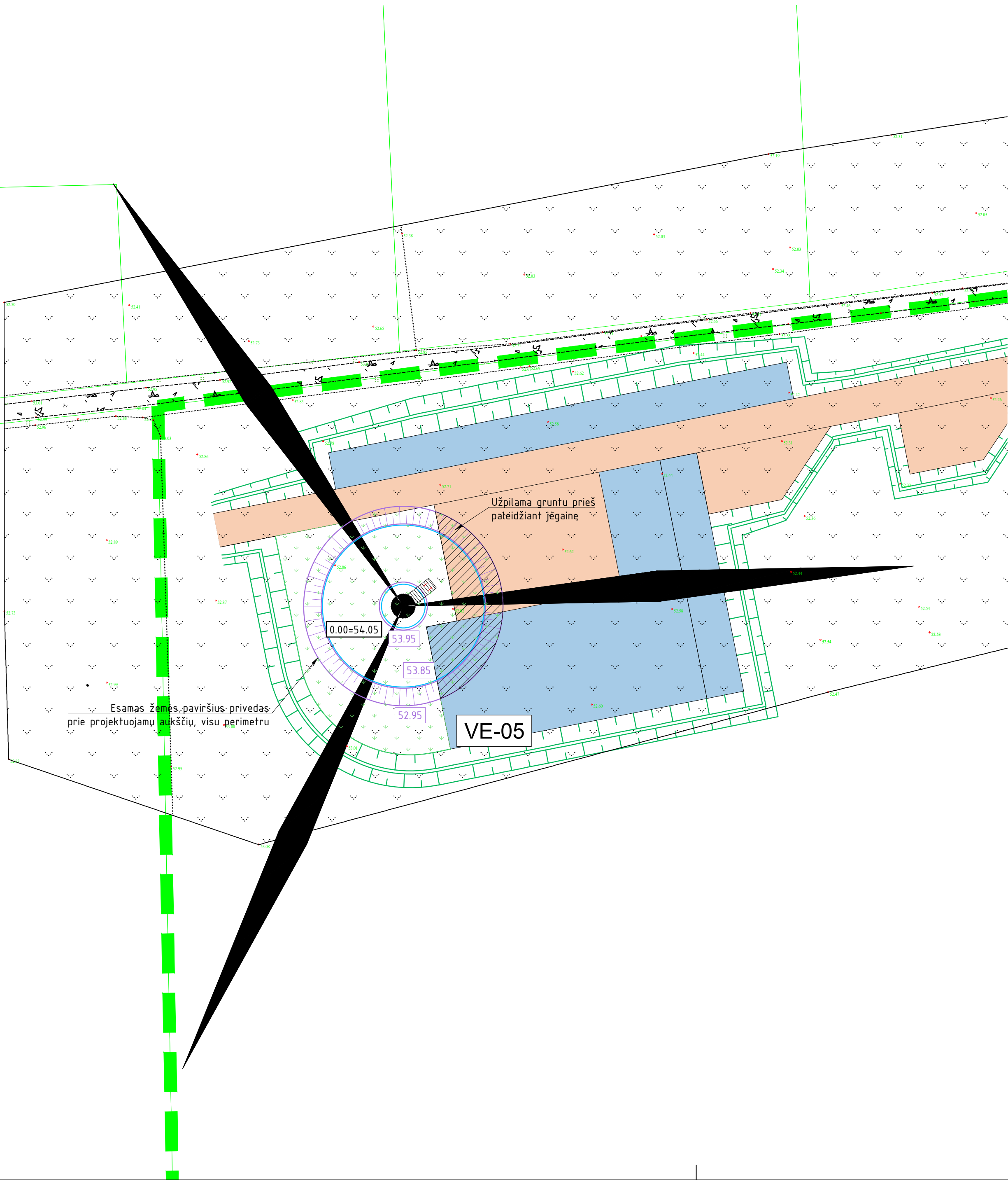
Sklypo aukščių planas M1:500
