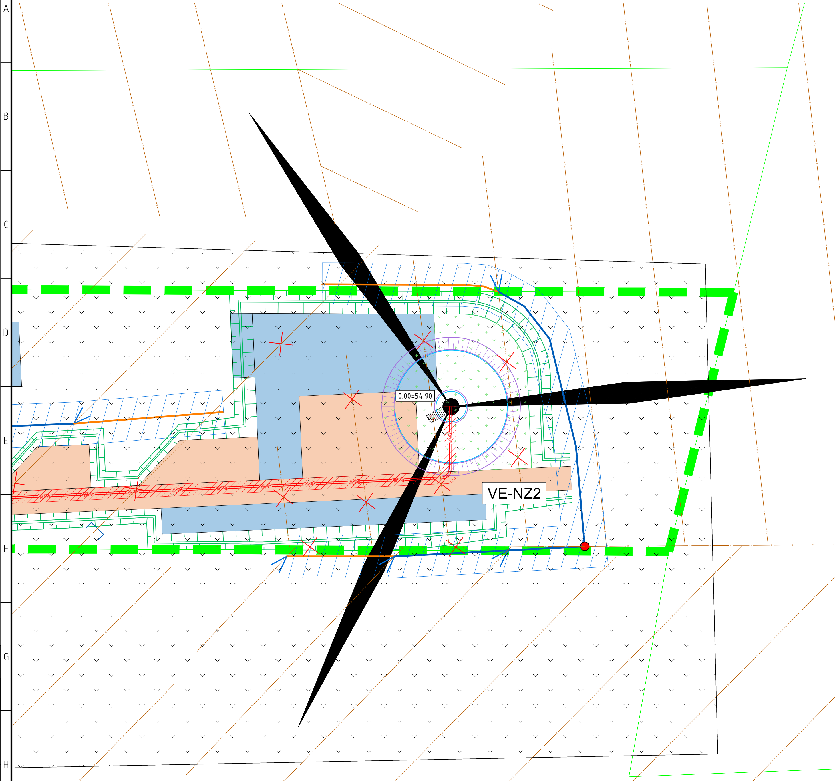
Sklypo inžinerinių tinklų planas M1:500
