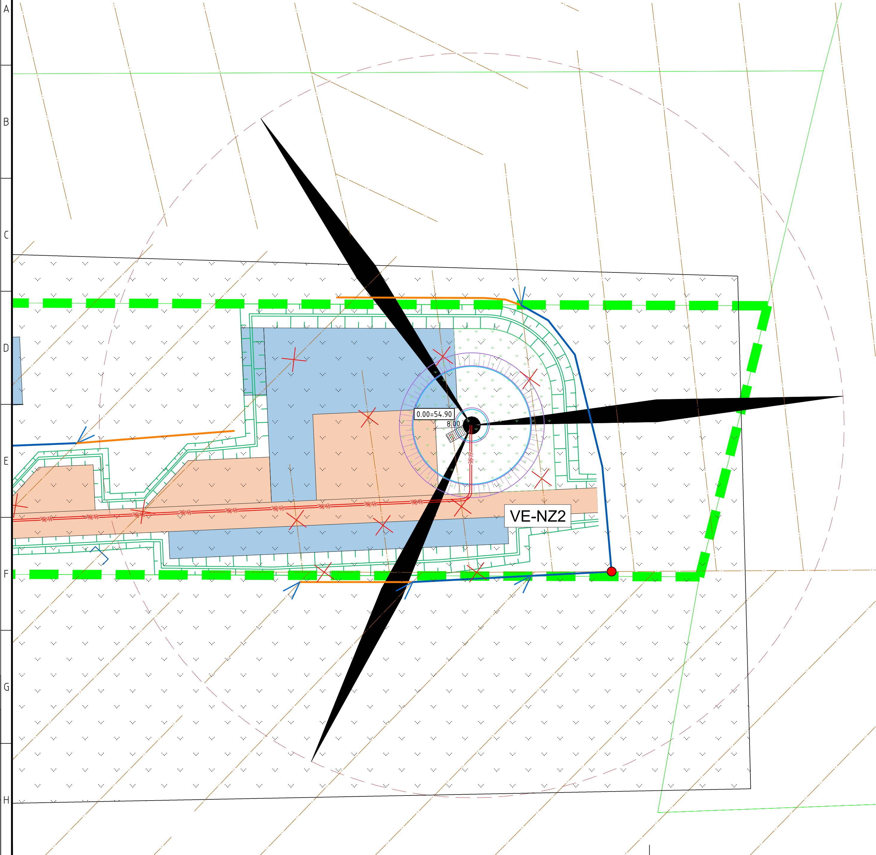
Sklypo planas M1:500
