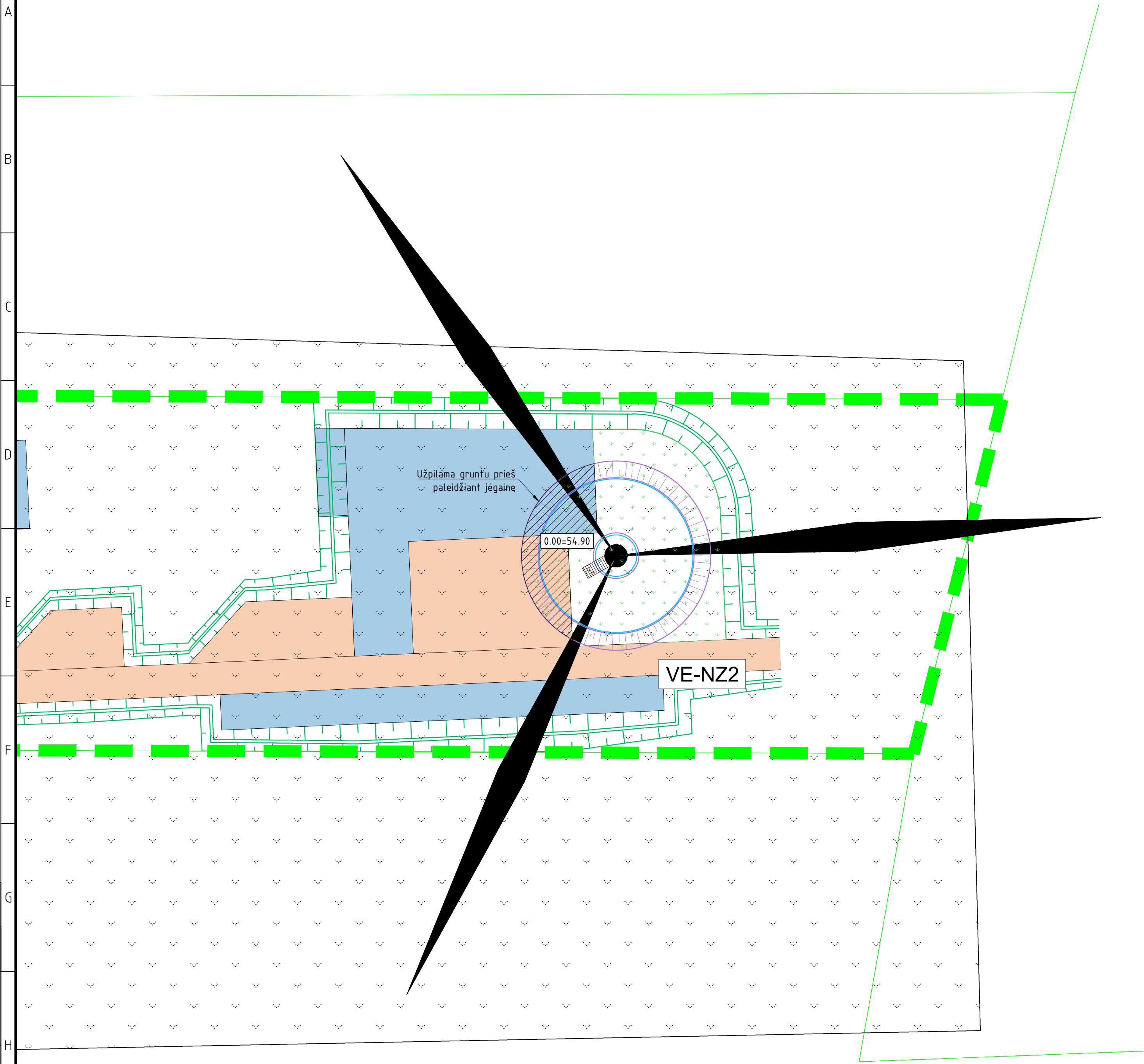
Sklypo sutrvarkymo planas M1:500
